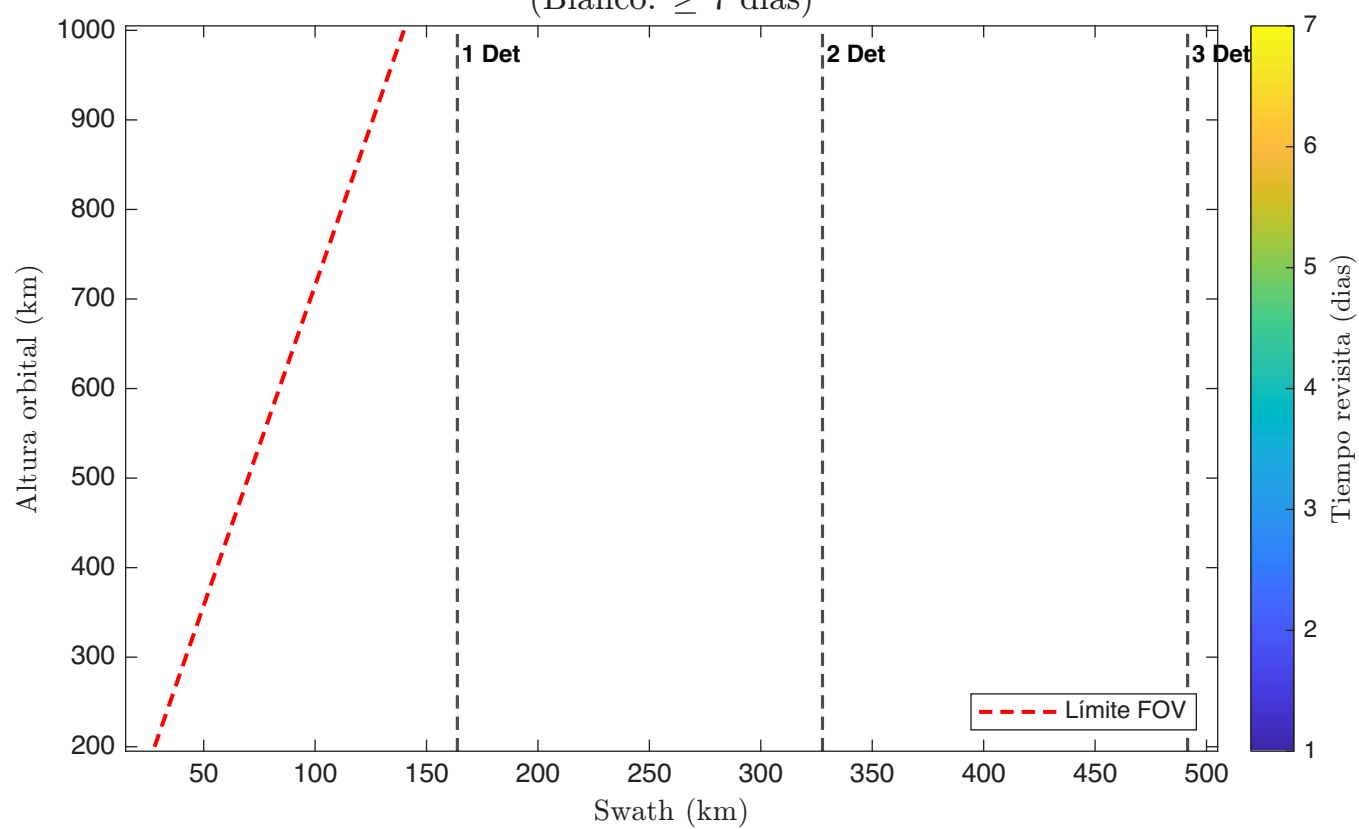
Tiempo Revisita - 2 Satellite(s); 1 Telescopio(s): TMA; Detector 2 (Blanco: \geq 7 dias)
